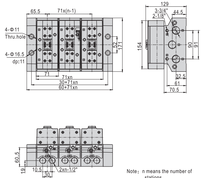
EAV430+ESV402M+ESV403M
