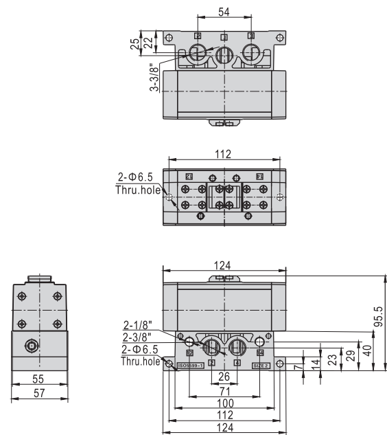
EAV330+ESV301M
