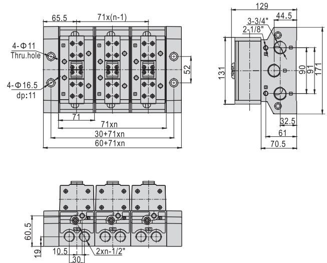
EAV430+ESV402M+ESV403M
